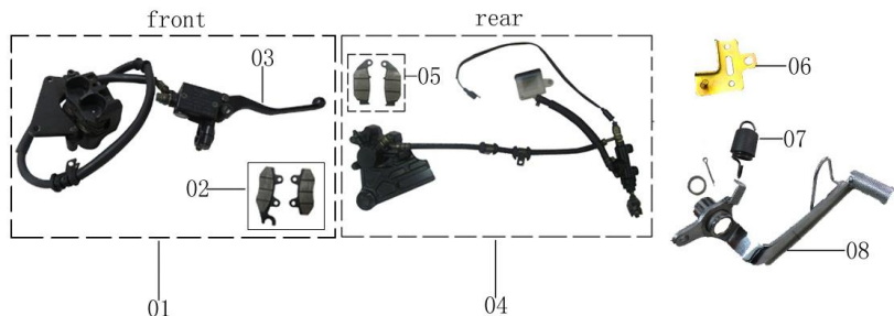
F-15 前后制动器 FRONT&REAR BRAKE
