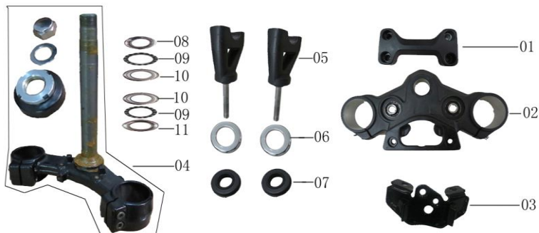
F-04 方向柱 STEERING STEM
