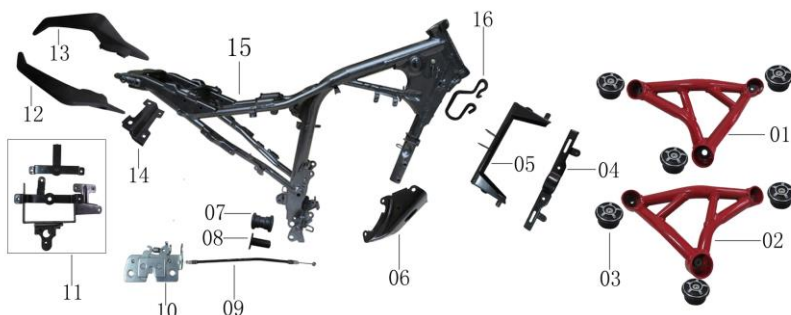
F-18 车架总成 FRAME BODY
